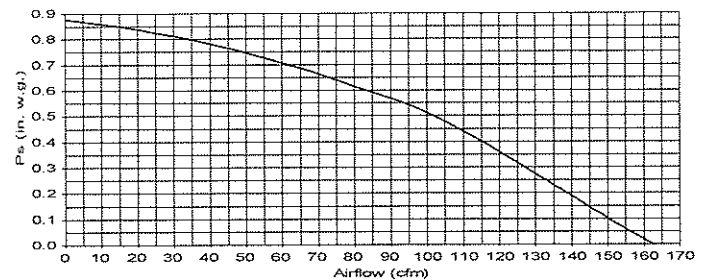
MODEL QTXE150FLT
