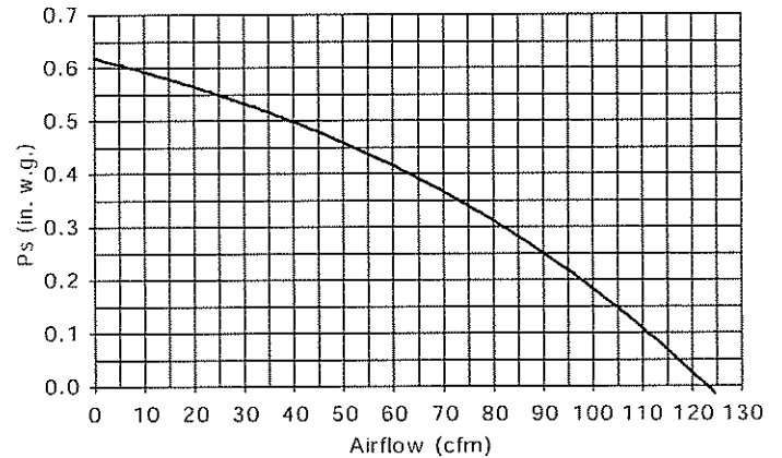
MODEL QTXE110FLT
