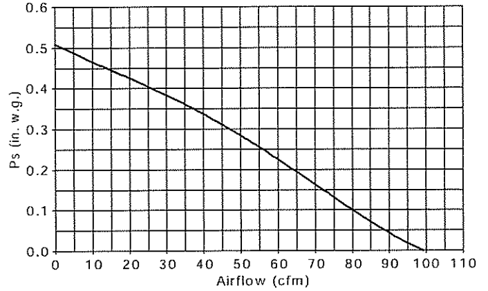
MODEL QTXE080FLT
